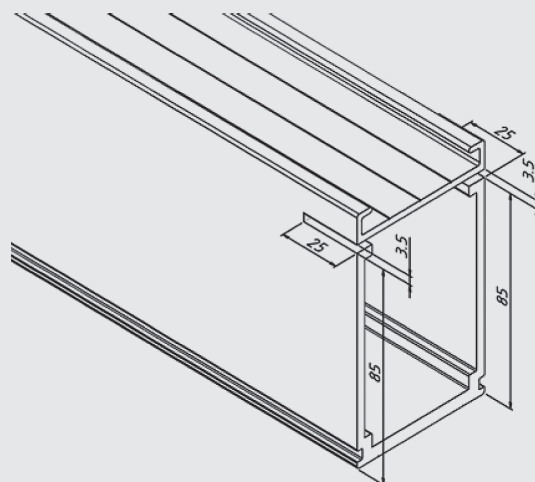
Einschnitte an den mittleren Tragprofilen zur Aufnahme des Blendprofils.
