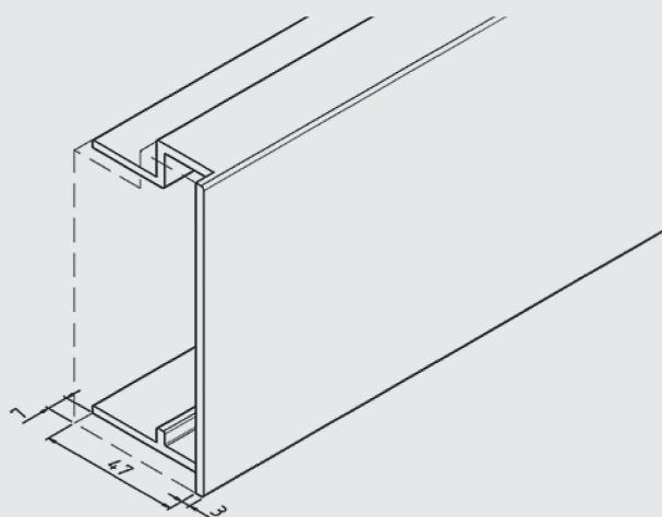
Einschnitte am Blendprofil für die Verbindung von Tragprofil und Blendprofil im Eckbereich.
