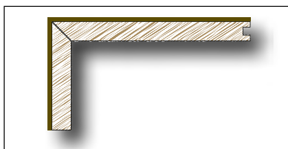
60131 Stirnschnitt ohne Sichtkante Coupe frontale sans bord visible
