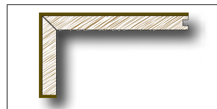
60132 Stirnschnitt mit Sichtkante Coupe frontale avec bord visible
