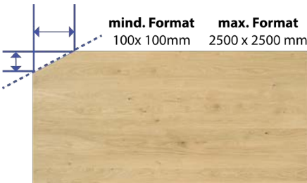
Winkelschnitt
